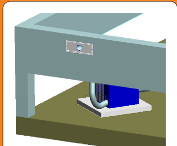
Kiinnitä poistoilmakanava poistopeltiin rakennuksen ulkopuolella.
