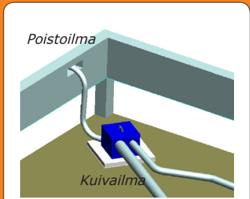
Asenna kuivailmakanavat ja poistoilmakanava kuvan mukaisesti
